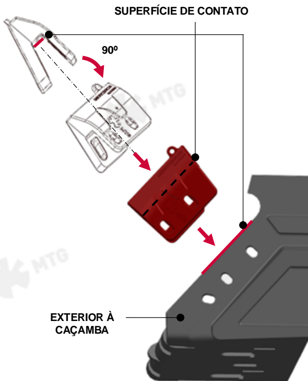
VISTA DE PERFIL DA CAÇAMBA
