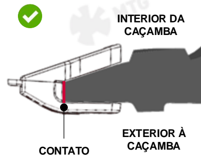
VISTA SUPERIOR DA CAÇAMBA
